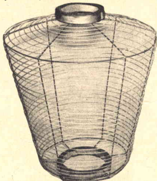
Fig. 4. - Gabbia in filo di ferro interamente saldata a stagno da ricoprirsi in finta pergamena e che costituisce il paralume della lampada.
