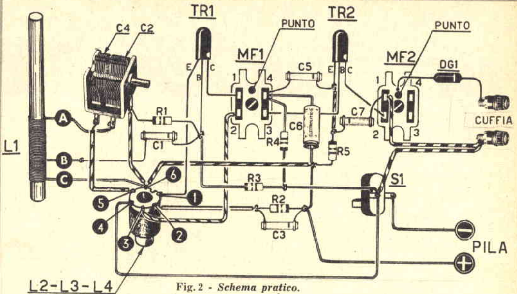
Fig. 2 - Schema pratico.
