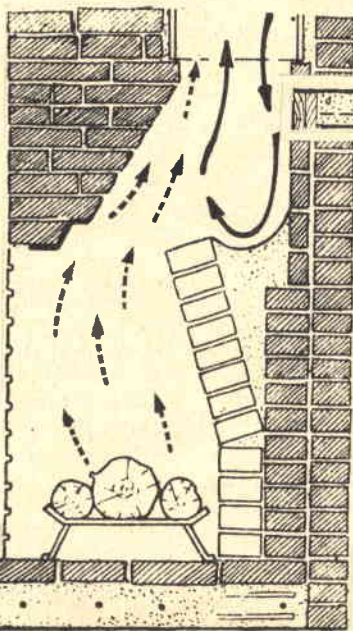
Fig. 5 - Il ferma-fumo risulta costituito da un rilievo a paratia in muratura, sistemato sulla parete di schiena del camino.
