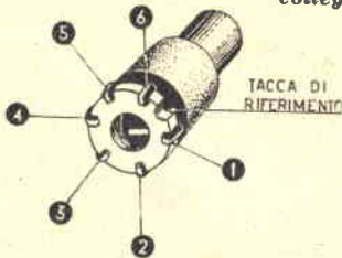
Fig. 4 - Bobina oscillatrice tipo Corbetta CS5. Per riconoscere l'ordine di successione dei vari collegamenti riferirsi alla tacca indicatrice.
