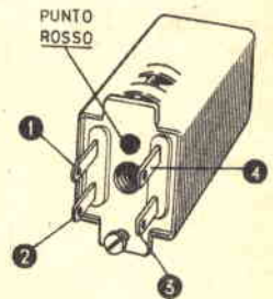
Fig. 4 - Bobina oscillatrice tipo Corbetta CS5. Per riconoscere l'ordine di successione dei vari collegamenti riferirsi alla tacca indicatrice.
