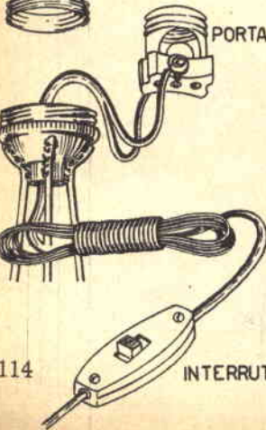
Fig. 3 - Particolari elettrici della lampada giapponese. Il portalam-pada in ottone è smontato nelle sue tre parti. L'interruttore volante rende comodo l'accendere e lo spegnere della lampada.
