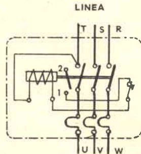
Fig. 2 - Teleruttore semplice.
