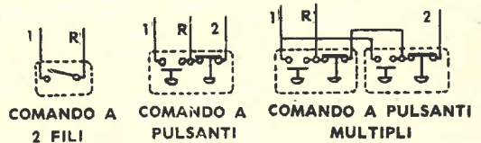
Fig. 2 - Teleruttore semplice.
