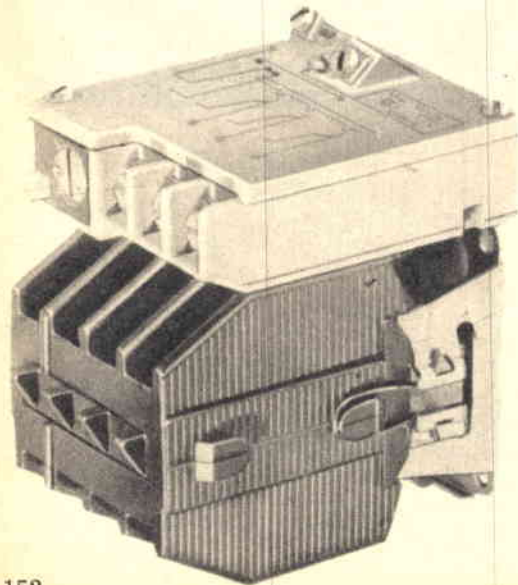
Fig.10 - Telesalvatore CORRADINI: — A) Involucro esterno - B) Schema elettrico - C) Complesso interno. Le apparecchiature della Società CORRADINI e PRIMAVESI di Milano sono costruite secondo le norme CEI e le norme di sicurezza ENPI. Sono semplici, precise e di lunga durata.
