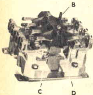
Fig. 8 - Istruzioni di montaggio dei contatti mobili del telesalvav motore della Società CORRADINI E PRIMAVERSI.
