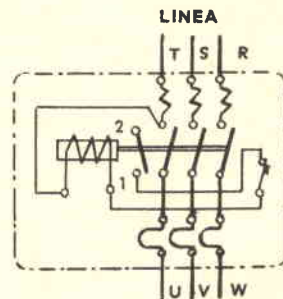
Fig. 3 - Teleruttore con relé termico.
